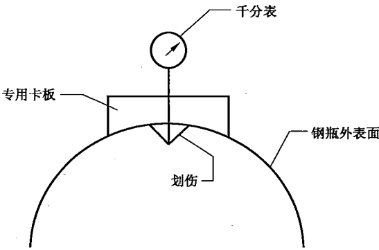
图 A.2 凹坑、磕伤、划伤深度的测量方法示意图
